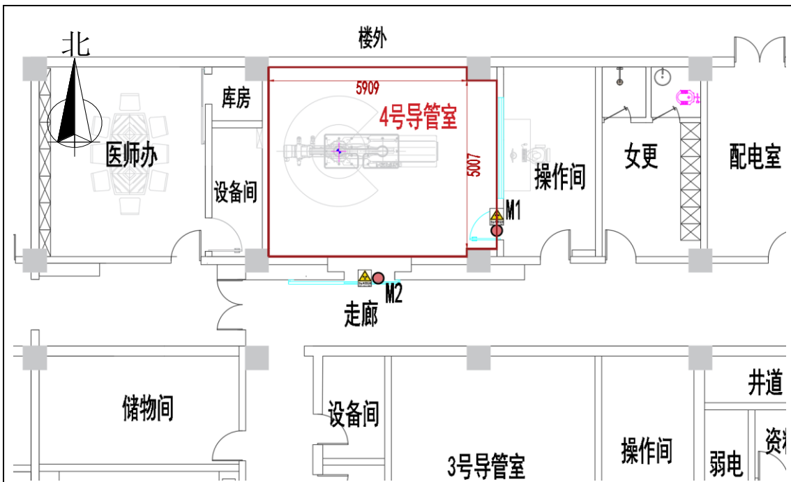
图 7-2 C 楼（住院楼）1 层 4 号导管室四周毗邻关系图（建成后）
