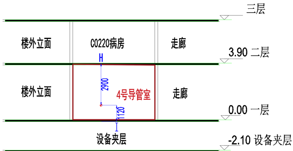
图 11-3 导管室楼上、楼下南北向剖面图
