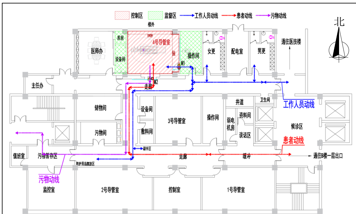
图 11-1 导管室分区和路由平面布局图
