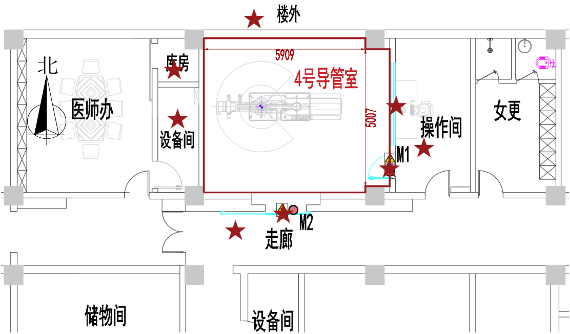
图 12-1 4 号导管室周围自行检测点位图（标注★为检测位置）
