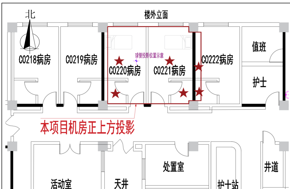
图 12-2 4 号导管室（楼上）自行检测点位图（标注★为检测位置）
