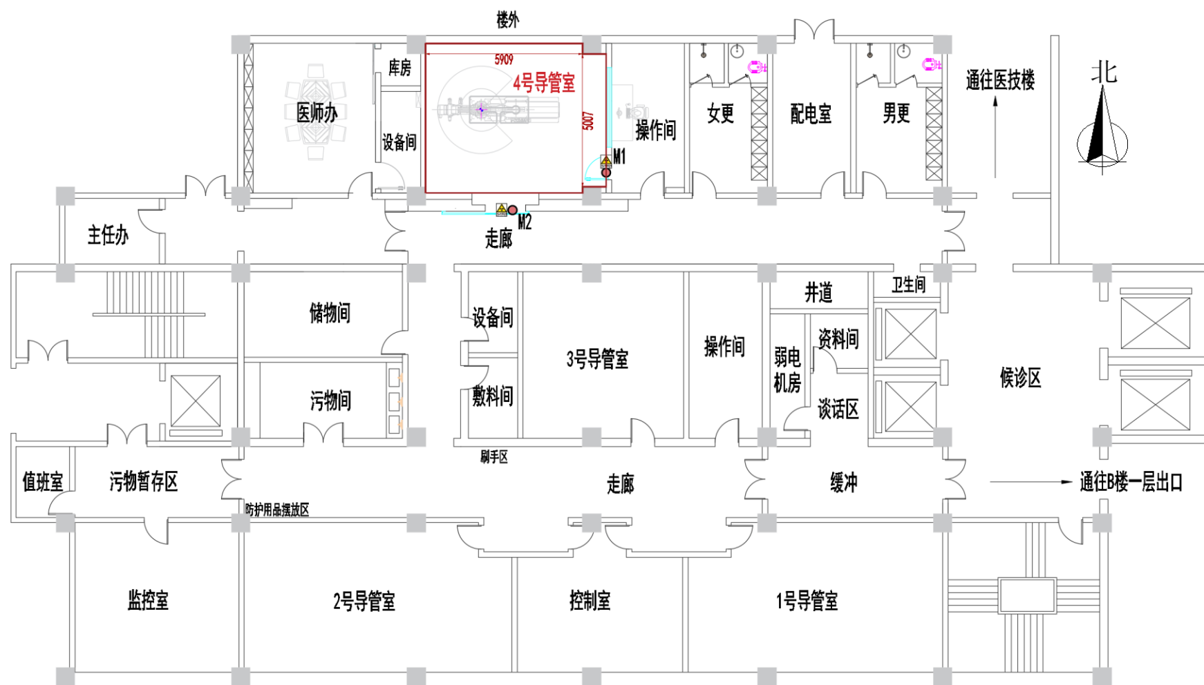
附图4 本部C楼（住院楼）1层4号导管室平面布局示意图（改造后）
