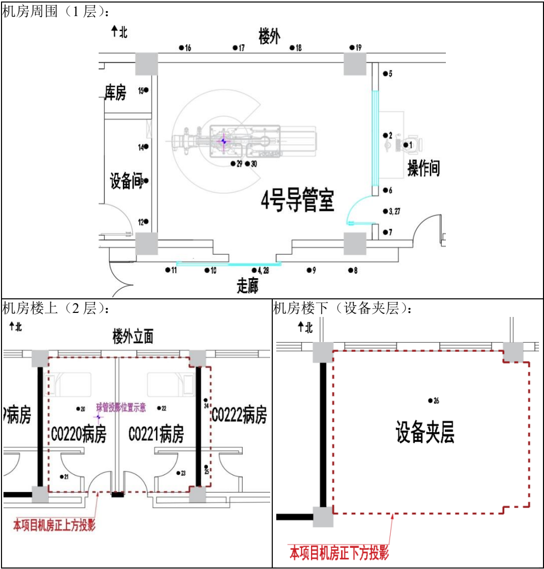
图 6-1 本部 4 号导管室防护验收检测示意图
